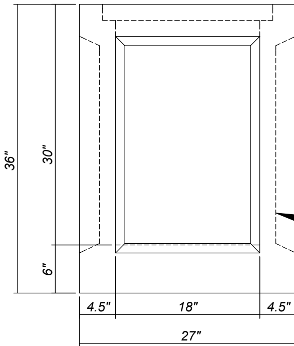
ELEVATION
